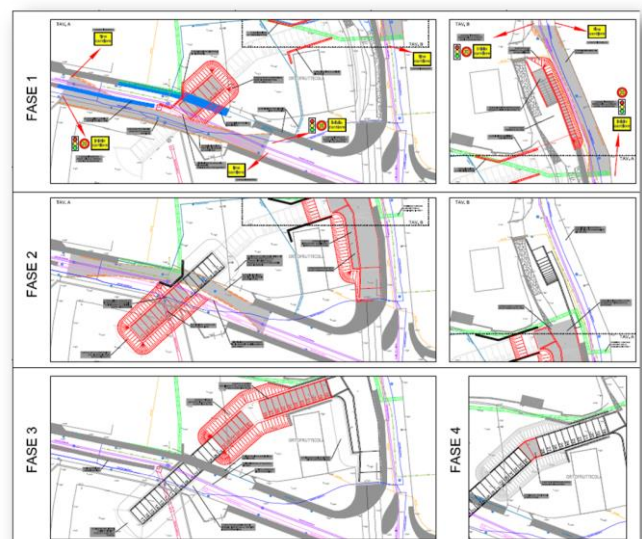
Studio delle fasi di cantiere.
