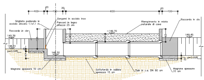
Particolare del progetto di un attraversamento.
