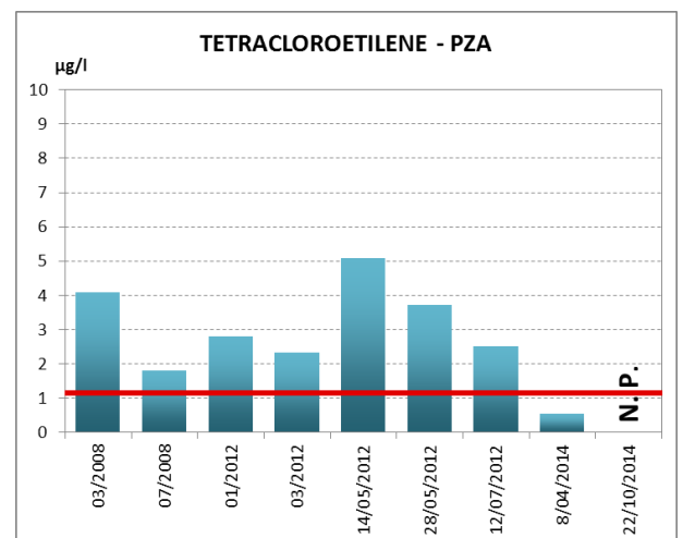
Esempio di analisi storiche delle concentrazioni di inquinante rilevate in determinati pozzi.
