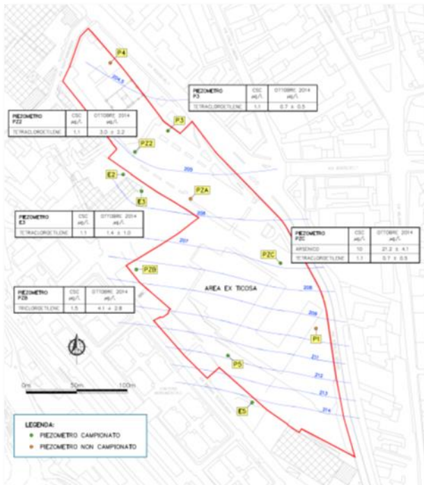
Planimetria dei campionamenti effettuati.
