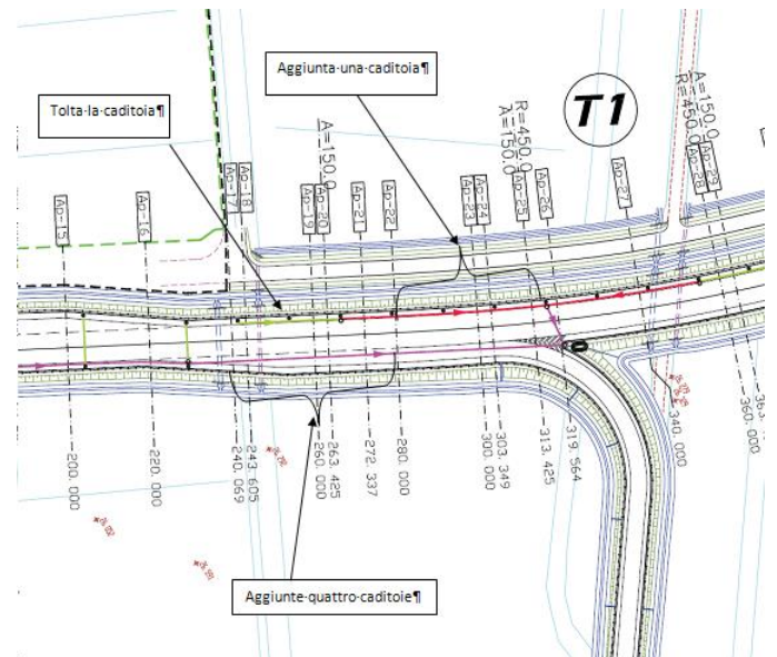
Dettaglio del progetto di dimensionamento del sistema di caditoie in variante al progetto in gara.
