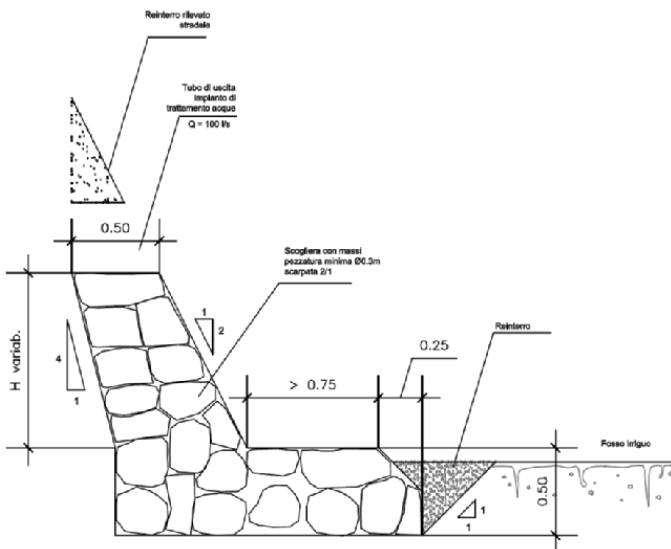
Disegno di una sezione tipologica.
